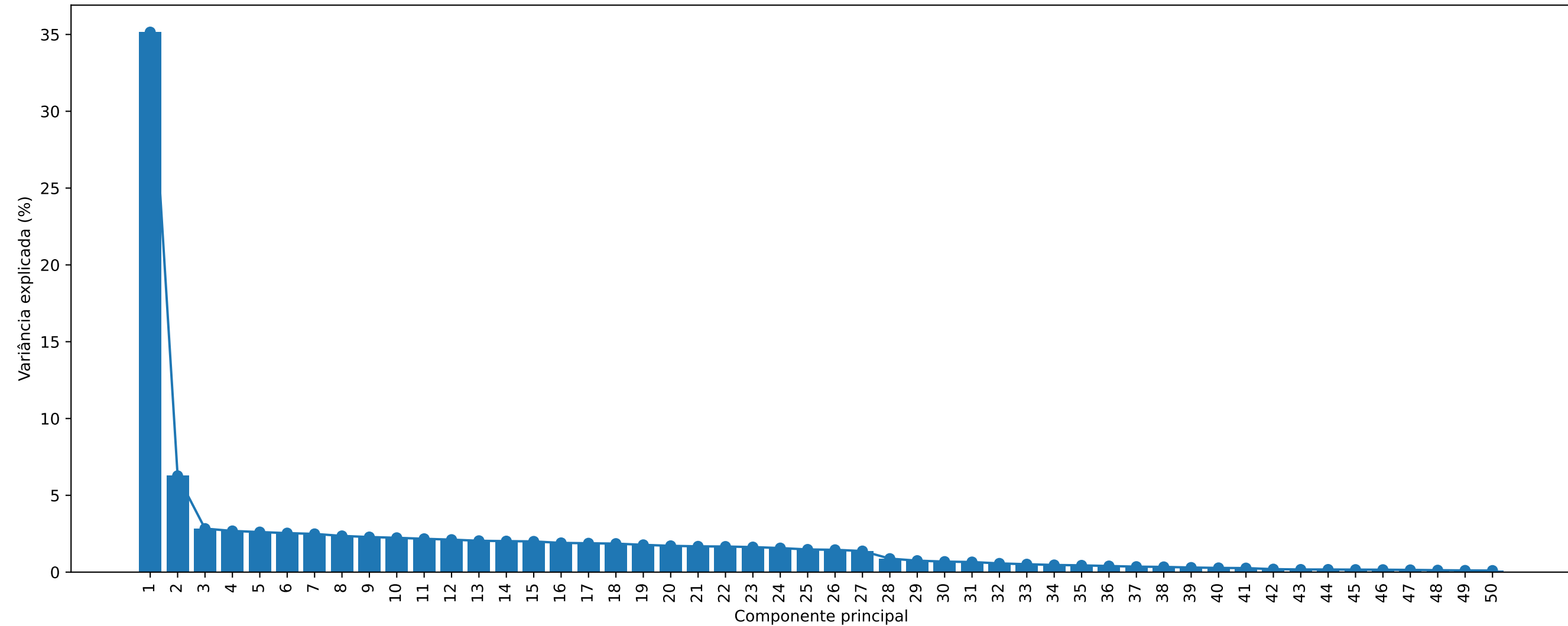
Scree Plot — Variância explicada por componente
